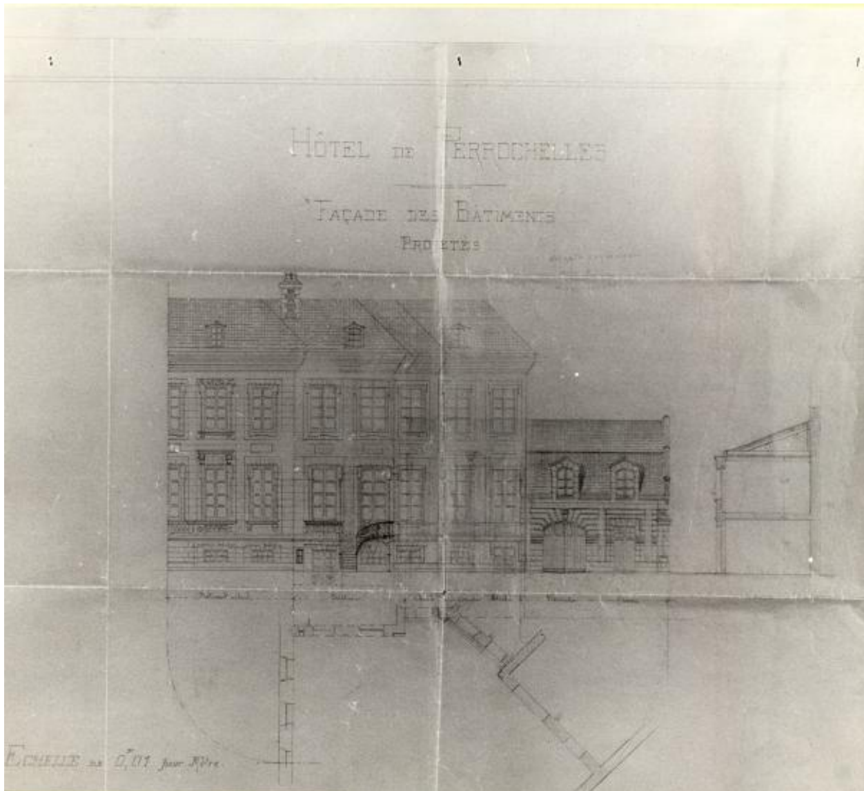
Aile droite, élévation interne, projet non réalisé, par l'architecte Auguste Martin, fin 19e siècle, éch. 1 : 100. (Collection particulière, M. Pousset).
