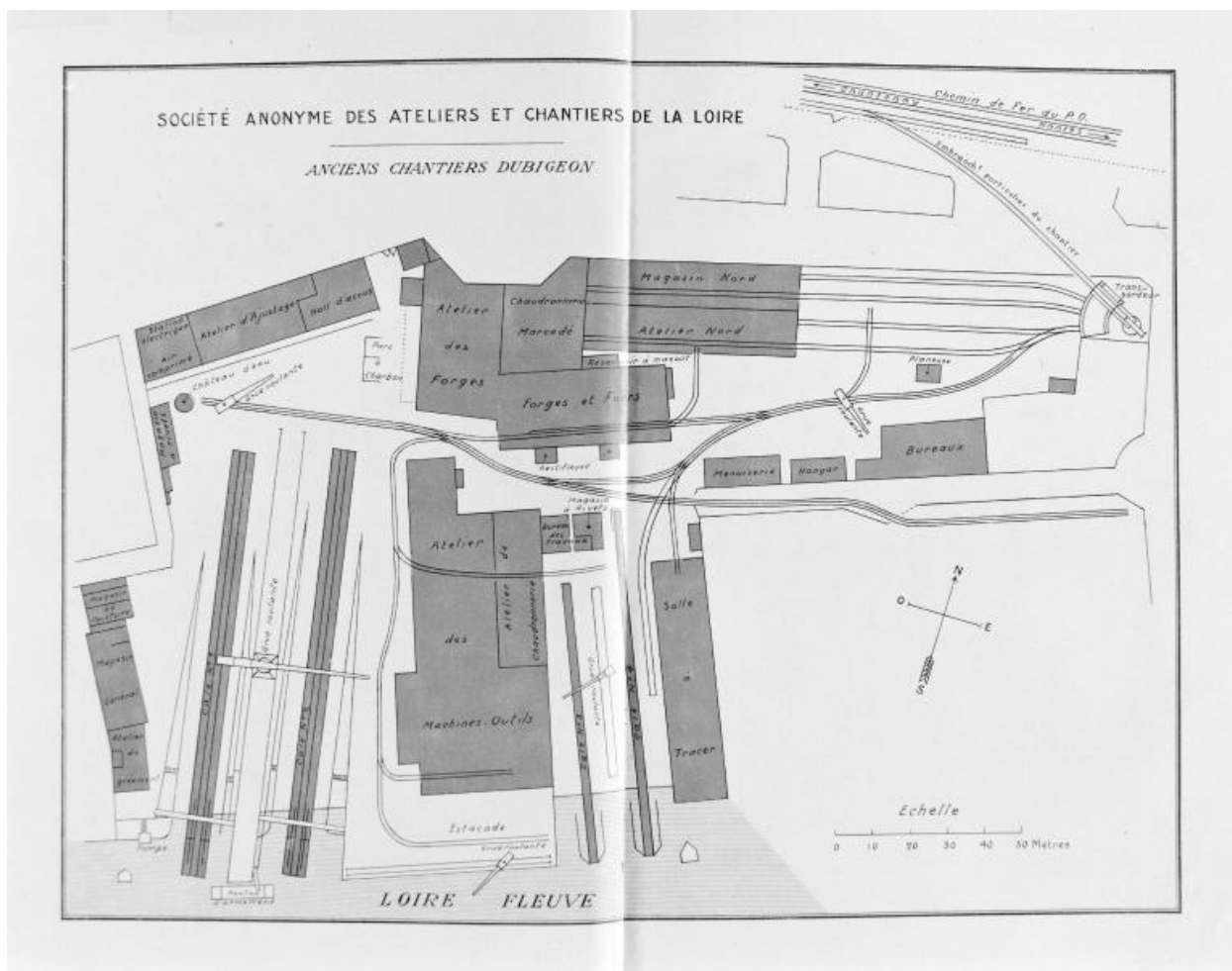
Plan des Anciens Chantiers Dubigeon, 1931.
