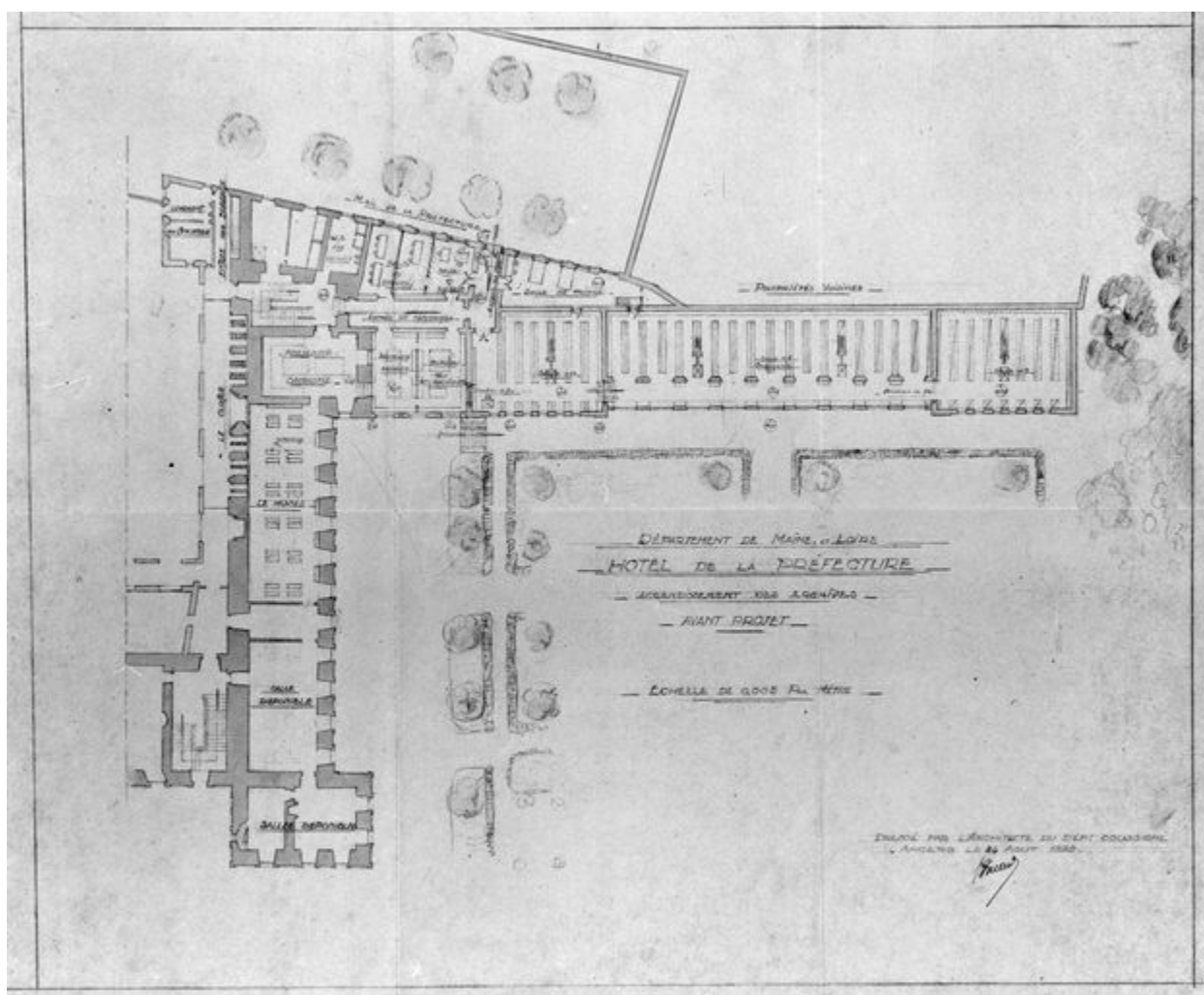
Département de Maine-et-Loire. Hôtel de la Préfecture. Agrandissement des Archives. Avant-projet : plan de l'aile est de l'abbaye Saint-Aubin et du nouveau bâtiment des Archives, par l'architecte du département Ernest Bricard, 1929. (Archives départementales de Maine-et-Loire ; N 1773).
