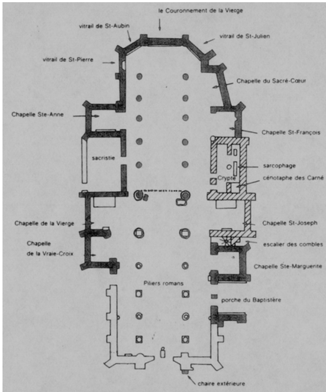
Plan d'ensemble.
