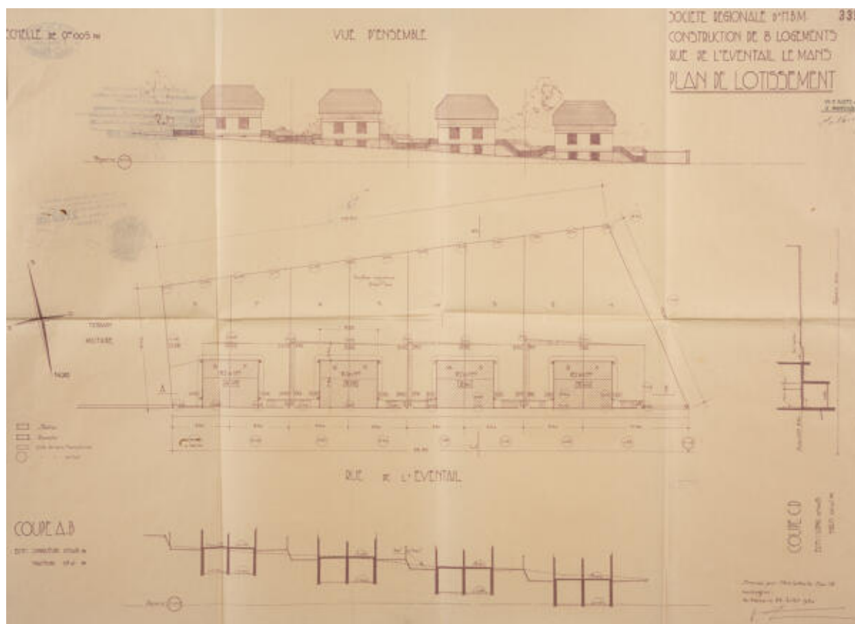
Plan général et élévation du permis de construire pour des maisons bon marché rue de l'Eventail, Paul Grosch.
