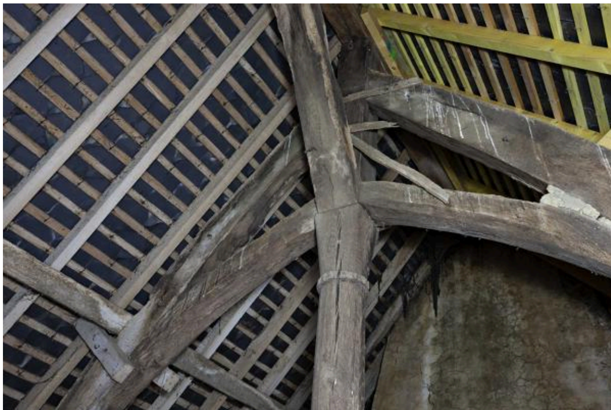
Charpente. Haut du poinçon et liens.
