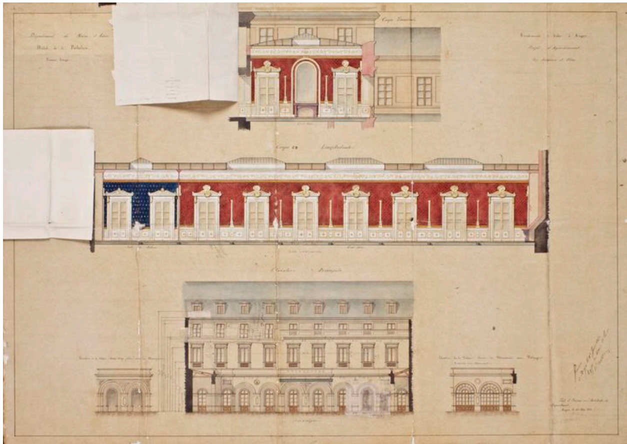
Coupes longitudinale et transversale de la salle des fêtes, projet, par l'architecte Ferdinand Lachèse, 1853. Dessin à la plume et aquarelle, éch. 1 : 100e. (Archives départementales de Maine-et-Loire ; N 1769).
