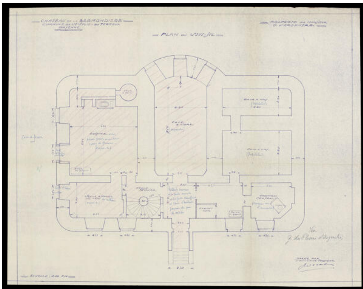
Plans de la reconstruction. Sous-sol.
