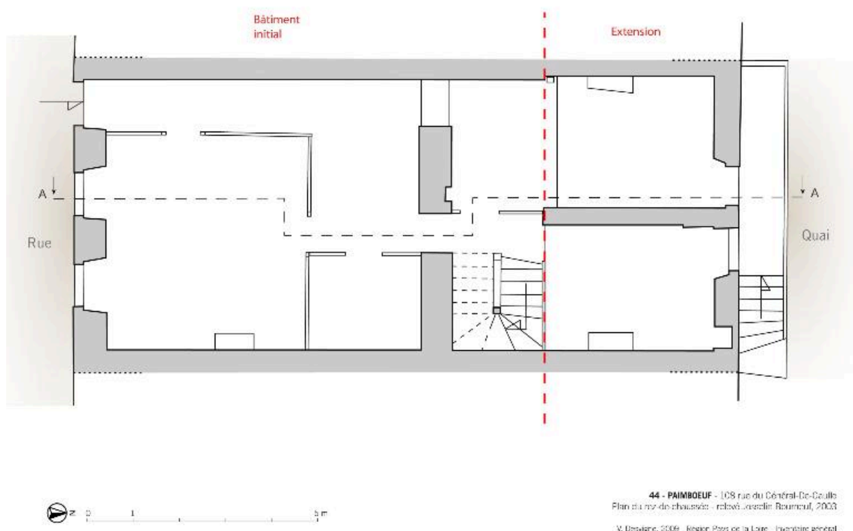
Maison, 108 rue du Général-De-Gaulle : plan du rez-de-chaussée.
