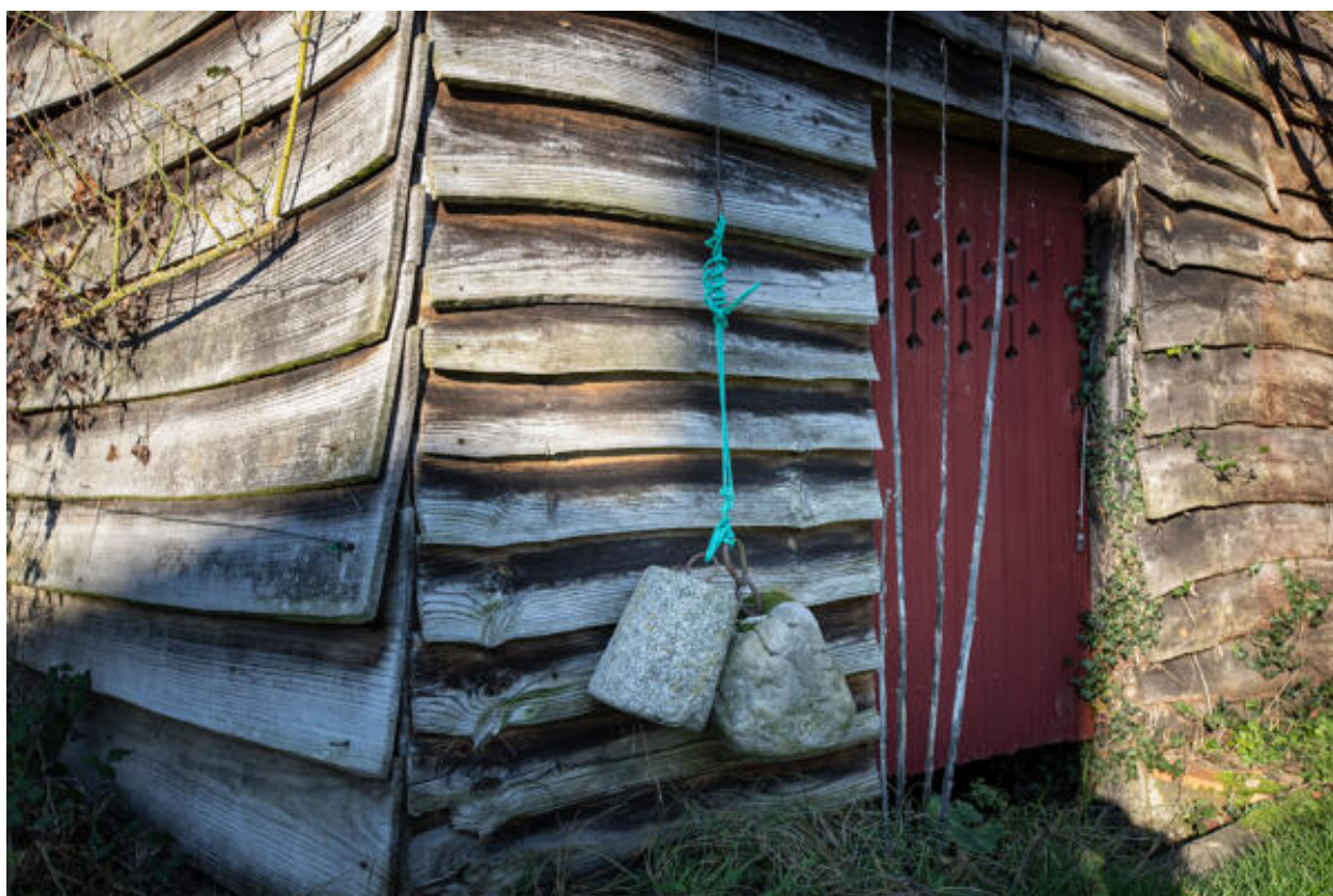
Ferme 2 : détail du bardage de la charretterie.
