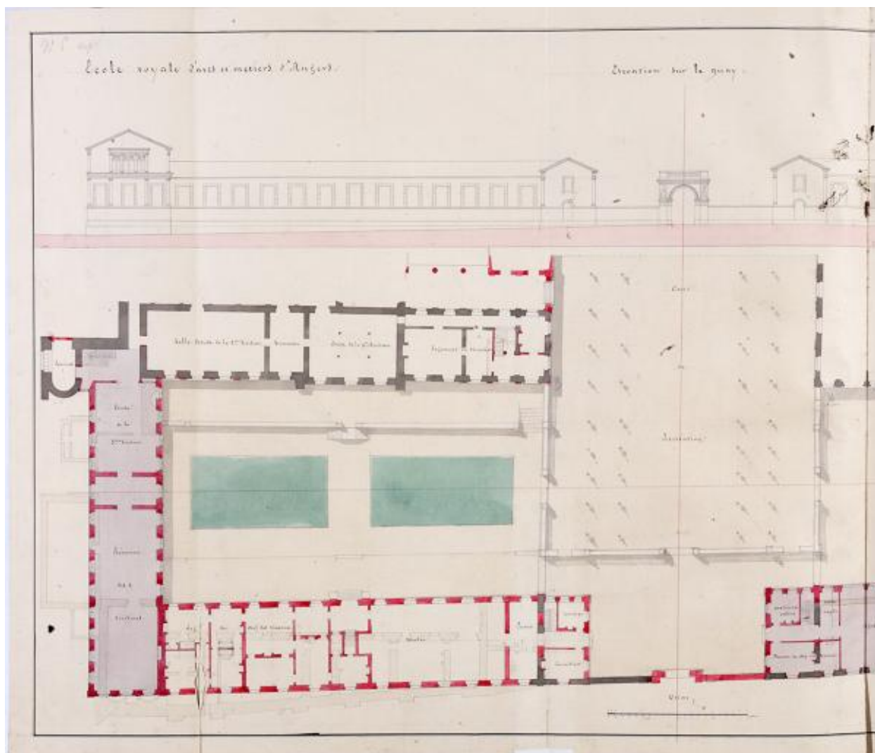
Ecole royale des Arts-et-Métiers d'Angers. Plan et élévation sur le quai, par Ch.-E. Isabelle, 1842. Détail : partie gauche de la planche. Parties à démolir en jaune et à construire en rouge.
