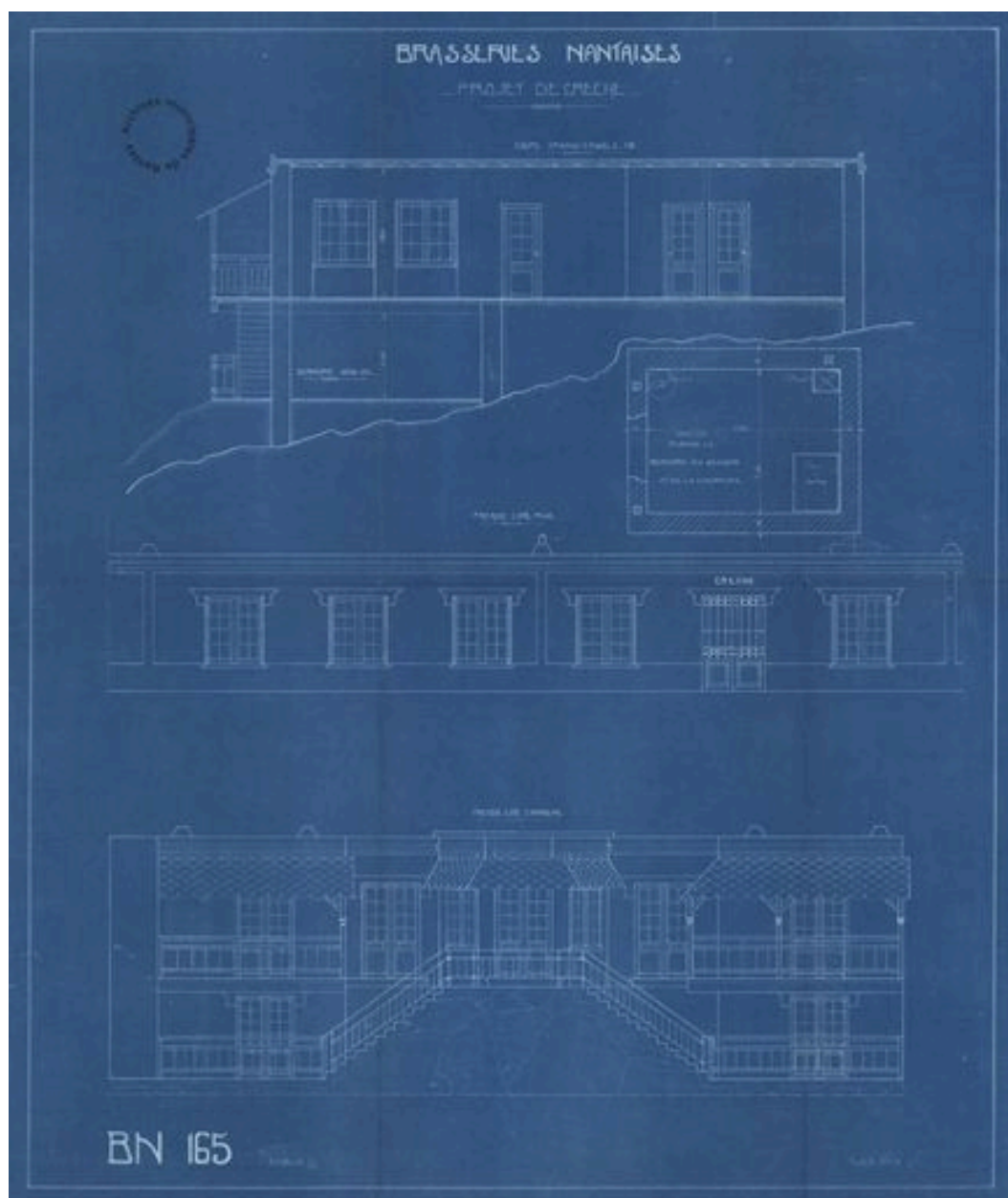
Elévations des crèches des Brasseries de la Meuse, 1928.
