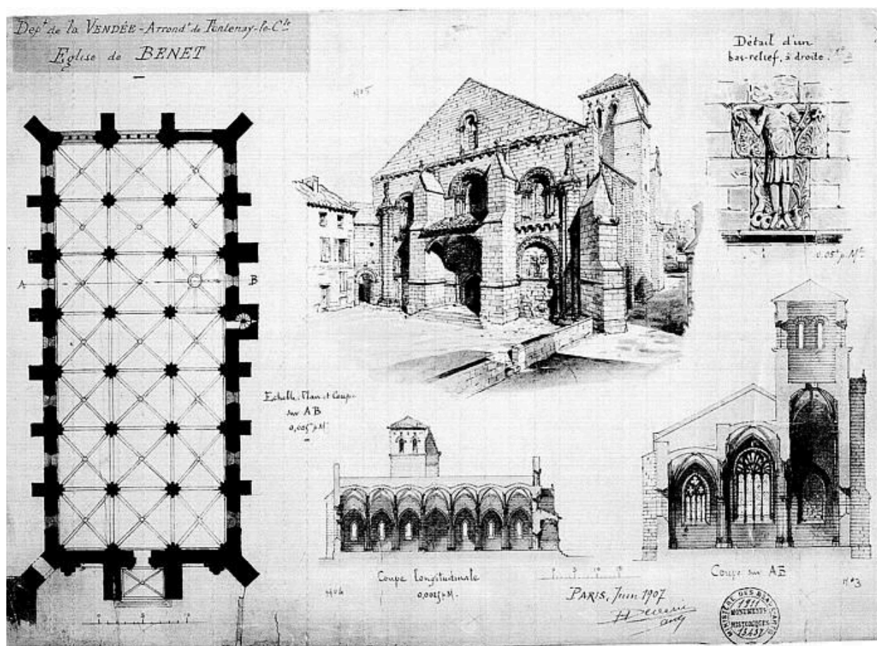
Plan, coupes et élévation de l'église de Benet en juin 1907 par H. Deverin.
