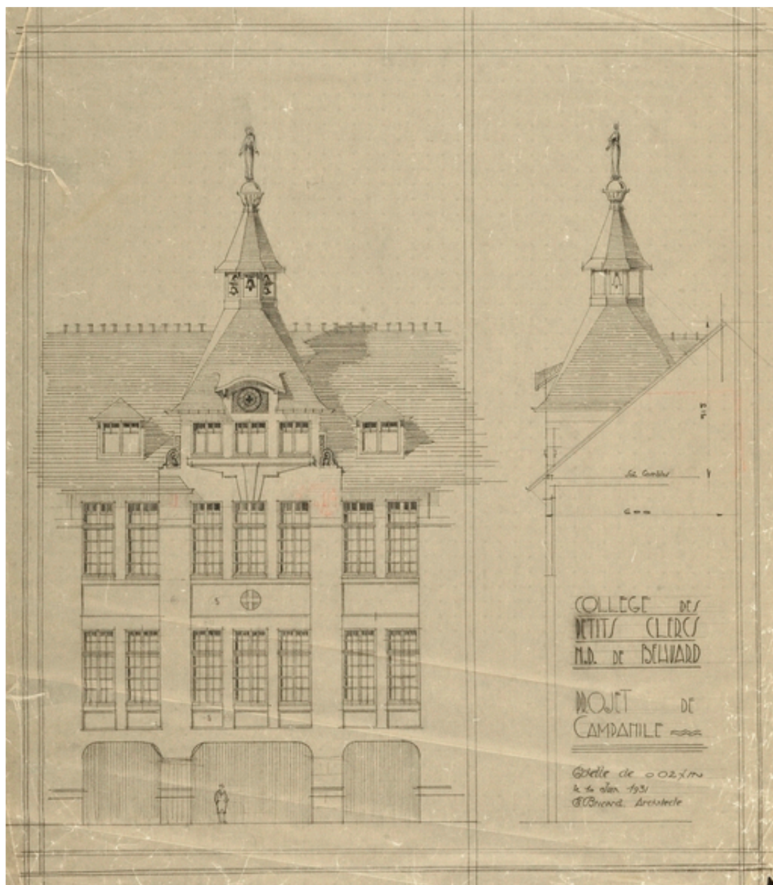
Collège des Petits Clercs de Notre-Dame de Béhuard. Projet de Campanile. Dressé par Ernest Bricard, le 10 juin 1931.
