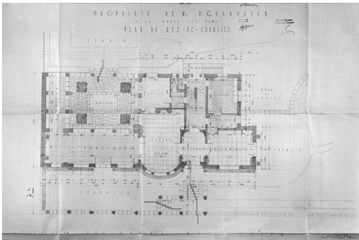
Plan du rez-de-chaussée au 1/50e de la villa Thuricia dressé pour M. Grandjean en 1938.
