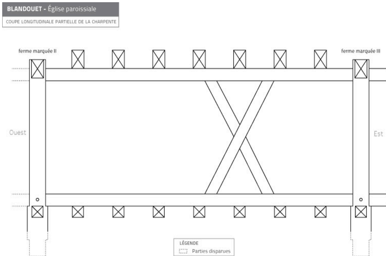
Coupe longitudinale partielle de la charpente.
