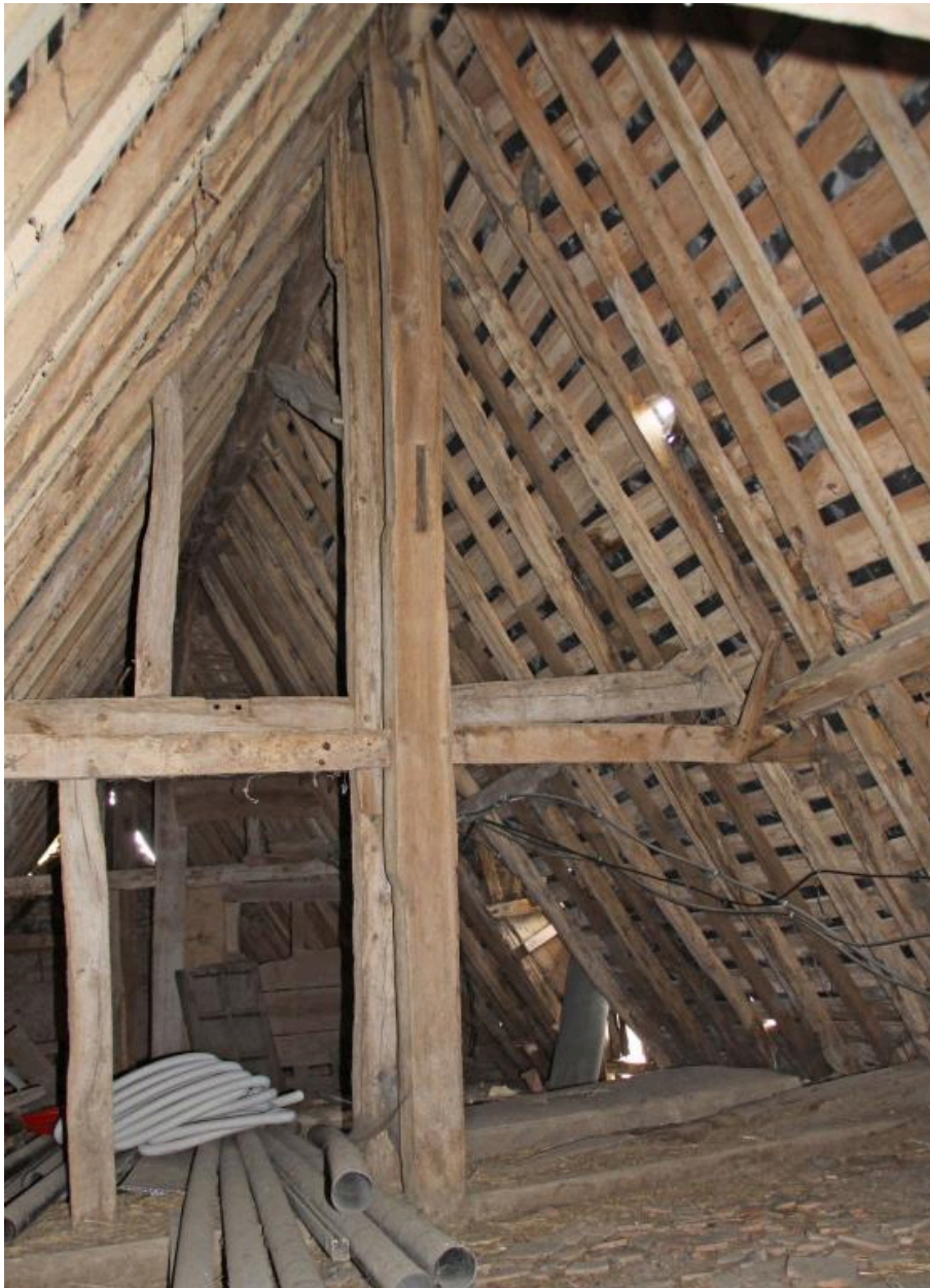
Comble : détail de la charpente (côté pignon maison-grange).
