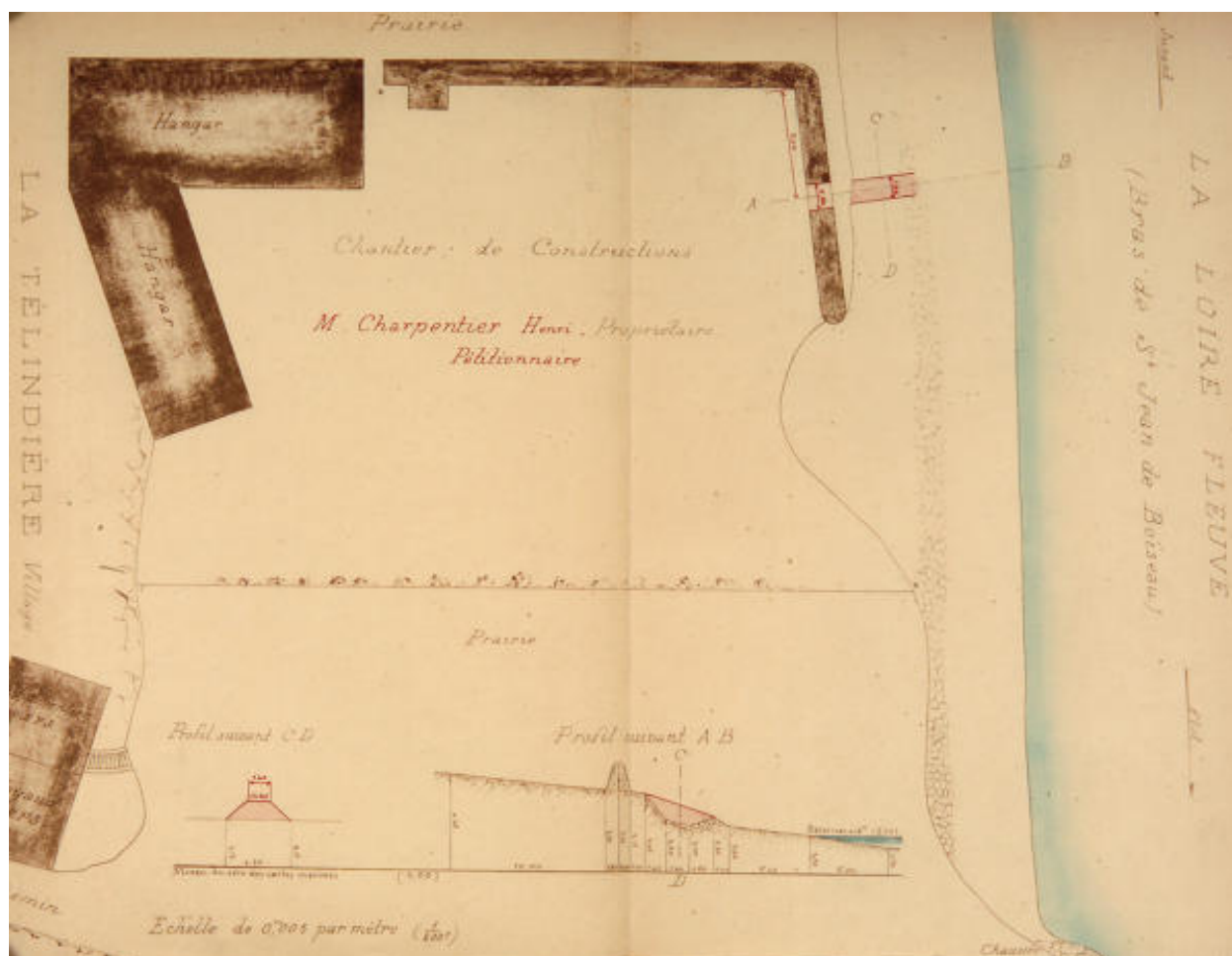
Chantier de construction navale. Pétition Charpentier. Plan et profil, 1906.
