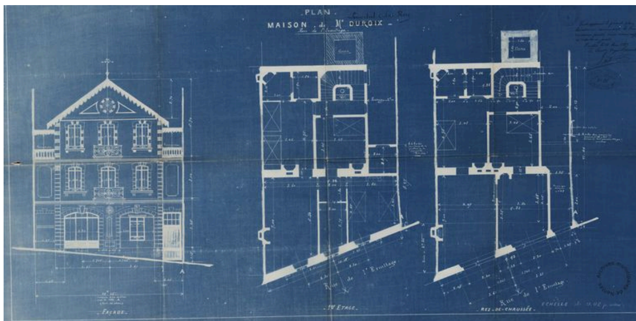
Plans et élévation de l'immeuble au 8 de la rue de l'Hermitage, 1856.
