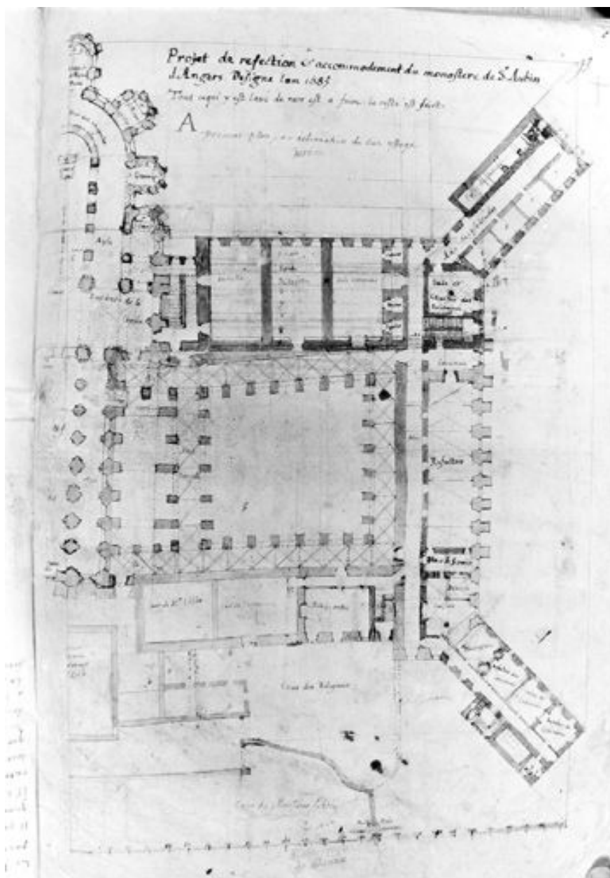
Projet "A" de 1685 : plan du rez-de-chaussée. ( Bibliothèque municipale de Meaux ; Ms. 44, f. 93).
