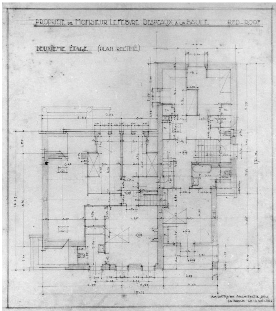
Plan du 2e étage au 1/50e de la villa Red-Roof pour M. Lefebvre Despeaux en 1926.
