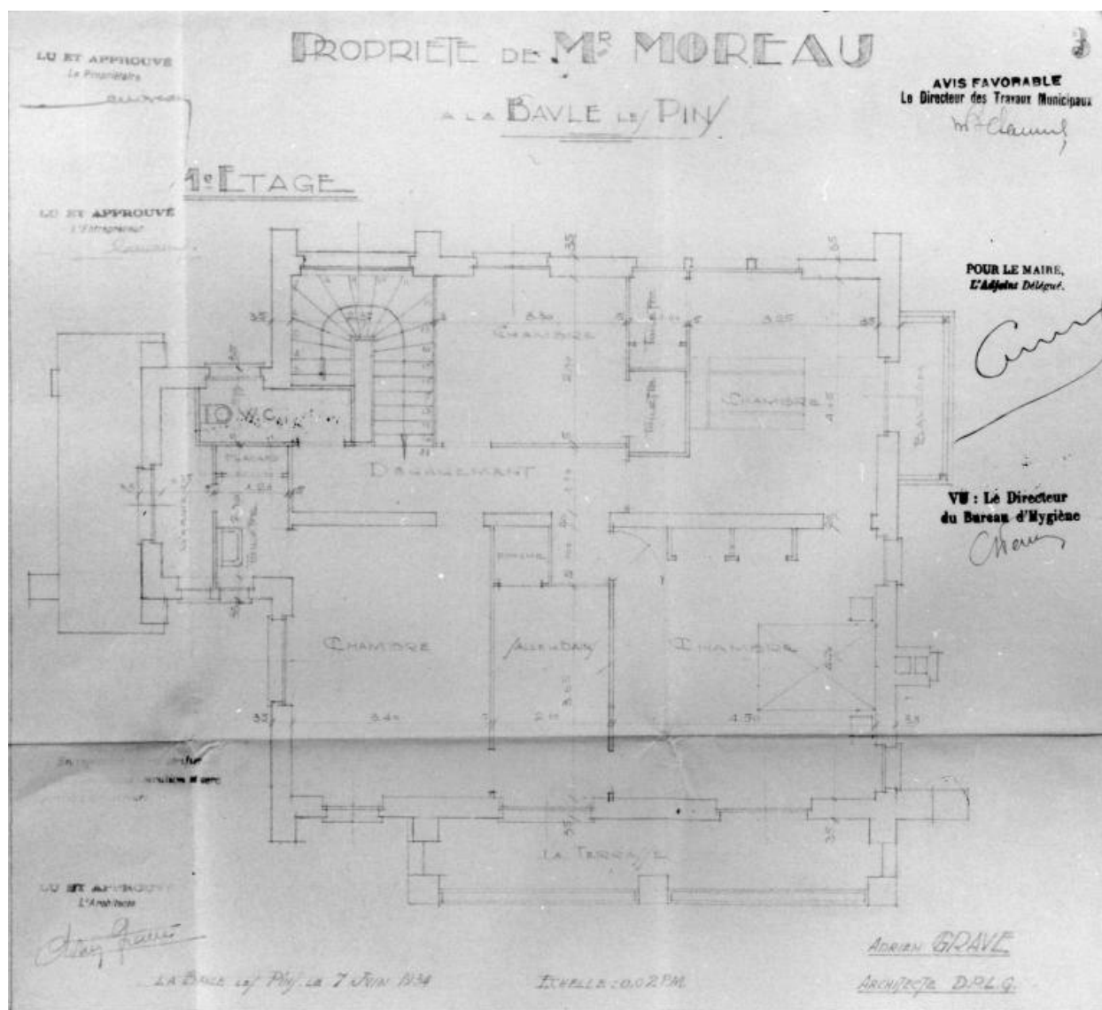
Plan du 1er étage au 1/50e de la villa Ohentzea dressé pour M. Moreau en 1934.
