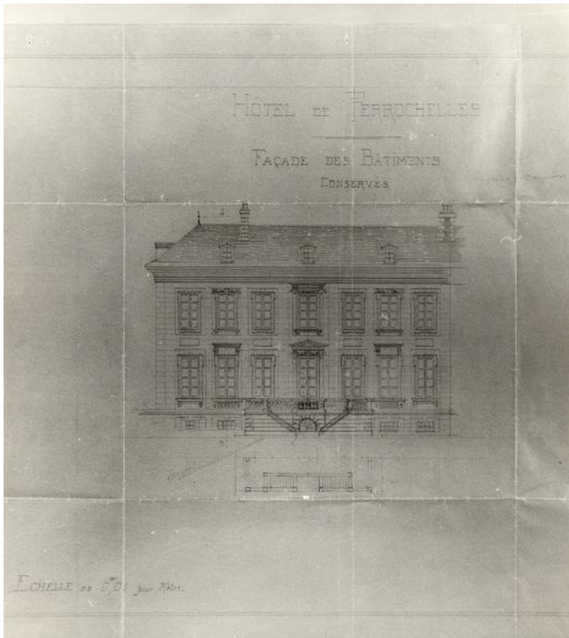
Elévation antérieure après remblaiement de la cour, projet, par l'architecte Auguste Martin. Dessin, fin 19e siècle, éch. 1:100e. (Collection particulière, Pousset).
