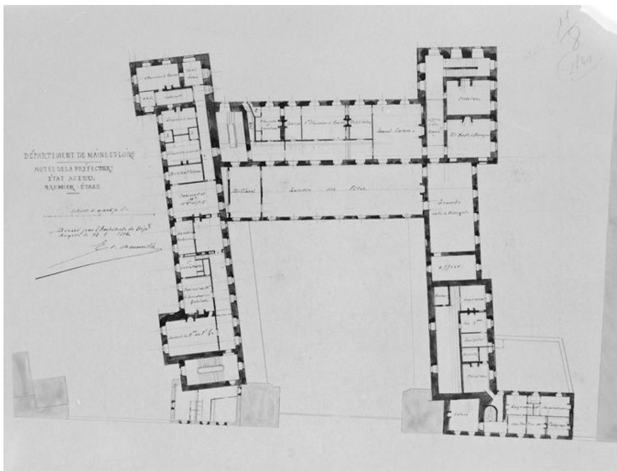
Département de Maine-et-Loire. Hôtel de la Préfecture. Etat actuel, 1er étage, dessin, par l'architecte Ernest Dainville, 1886. (Archives départementales de Maine-et-Loire ; 90 J 186 cote définitive).
