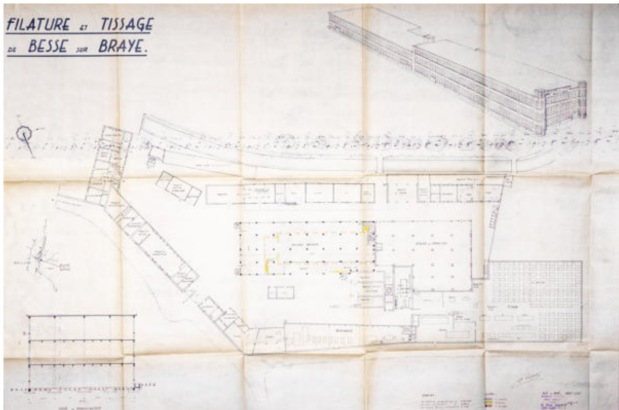
Plan, coupe et vue cavalière de construction des nouveaux ateliers de confection de l'usine de 1950.
