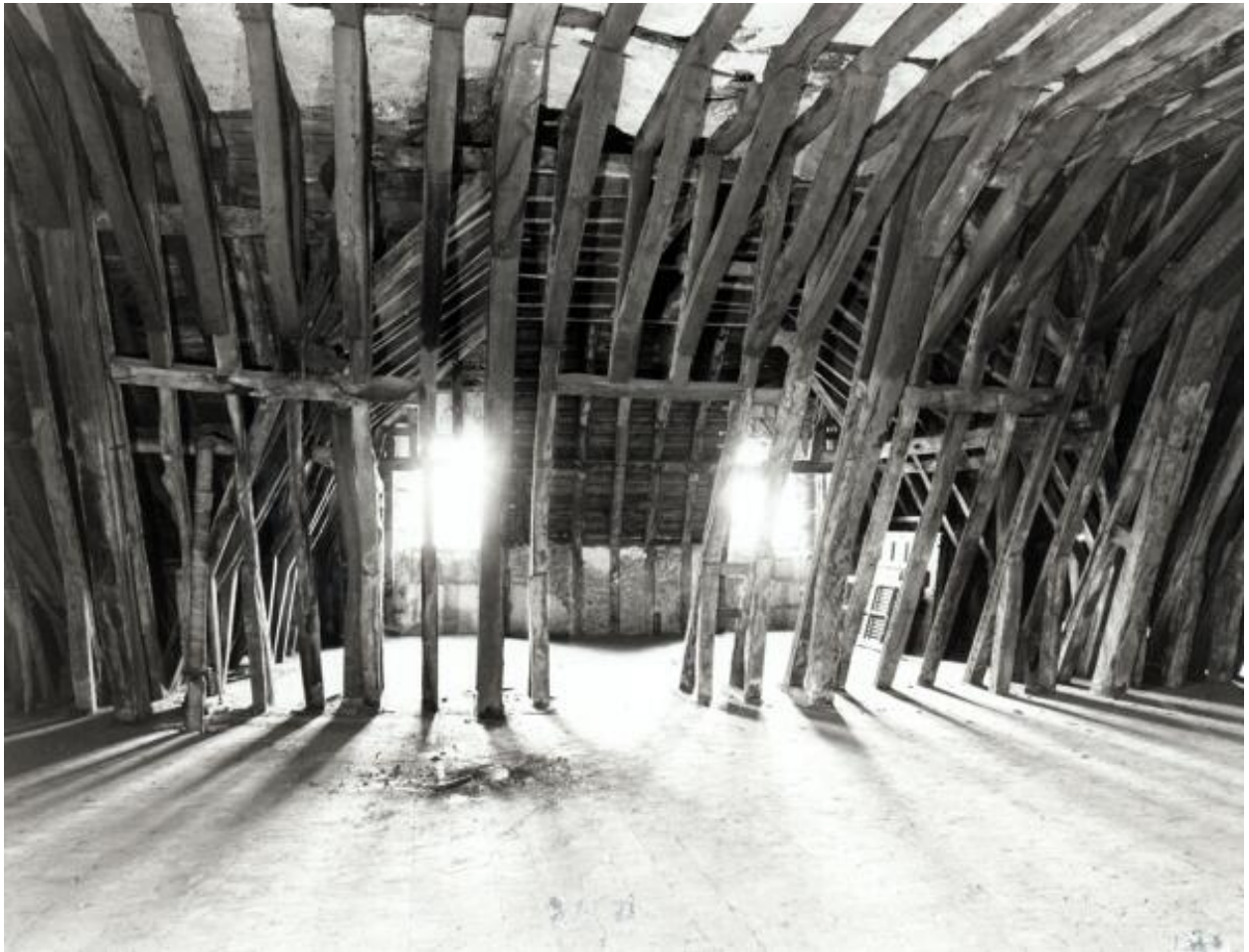
Aile ouest du cloître, étage de comble, charpente : vue transversale en axe ouest-est, vers l'une des croupes à double lucarnes.
