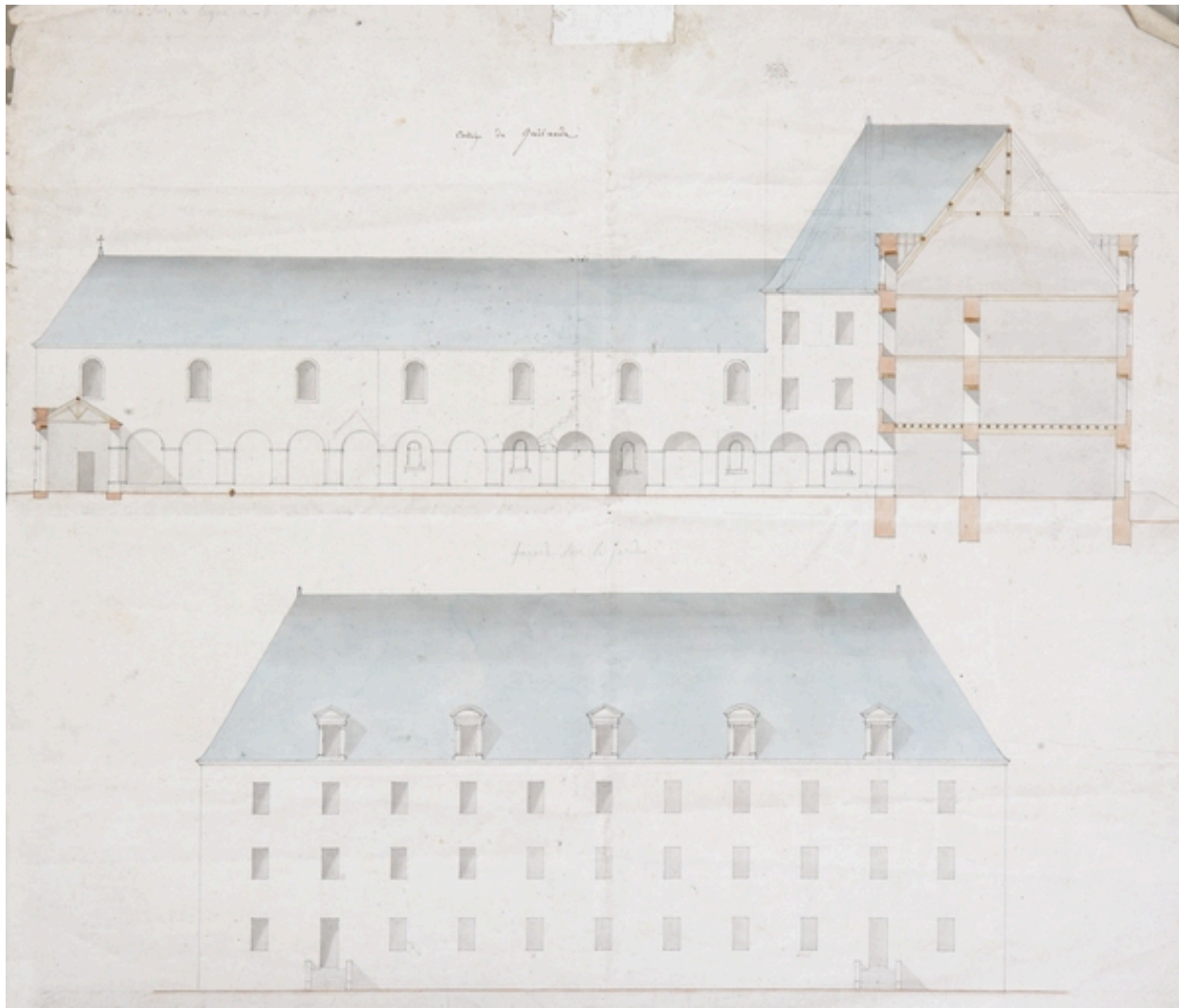
Élévation et coupe de l'aile nord par Henri Gilée, architecte, 2e moitié XIXe siècle.
