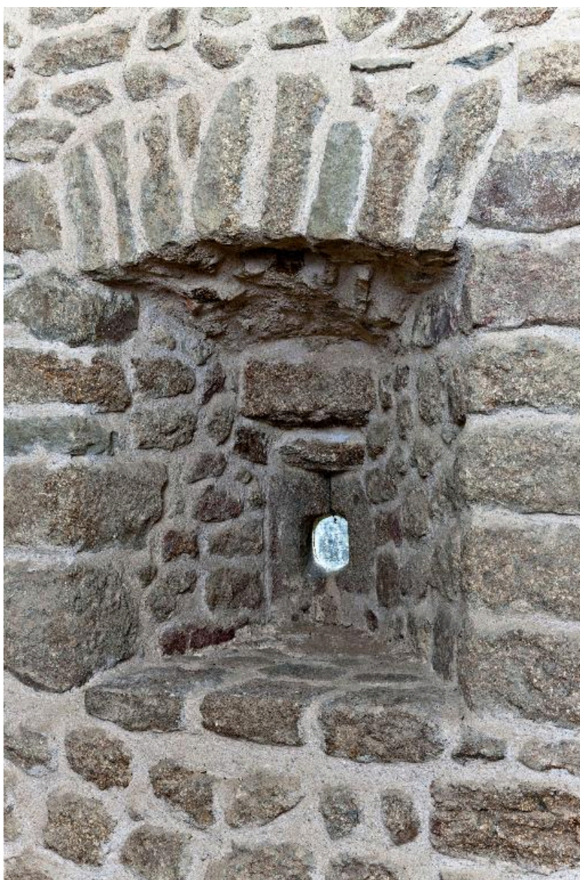
Premier étage de la tour nord : l'ouverture de tir (canonnière) ouest.
