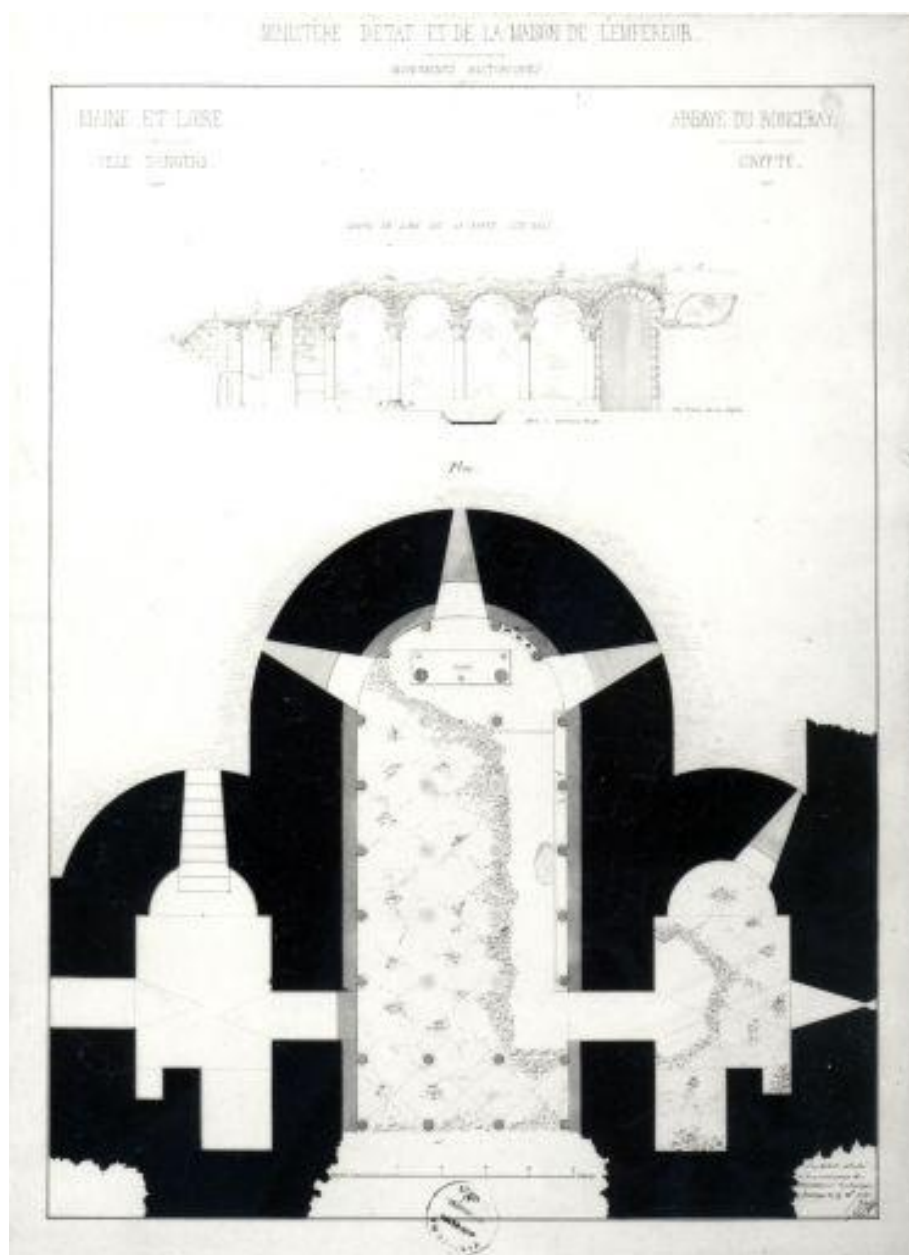
Plan d'ensemble de la crypte et coupe longitudinale vers sud de la chapelle centrale, par Ch. Joly-Leterme, 1857.
