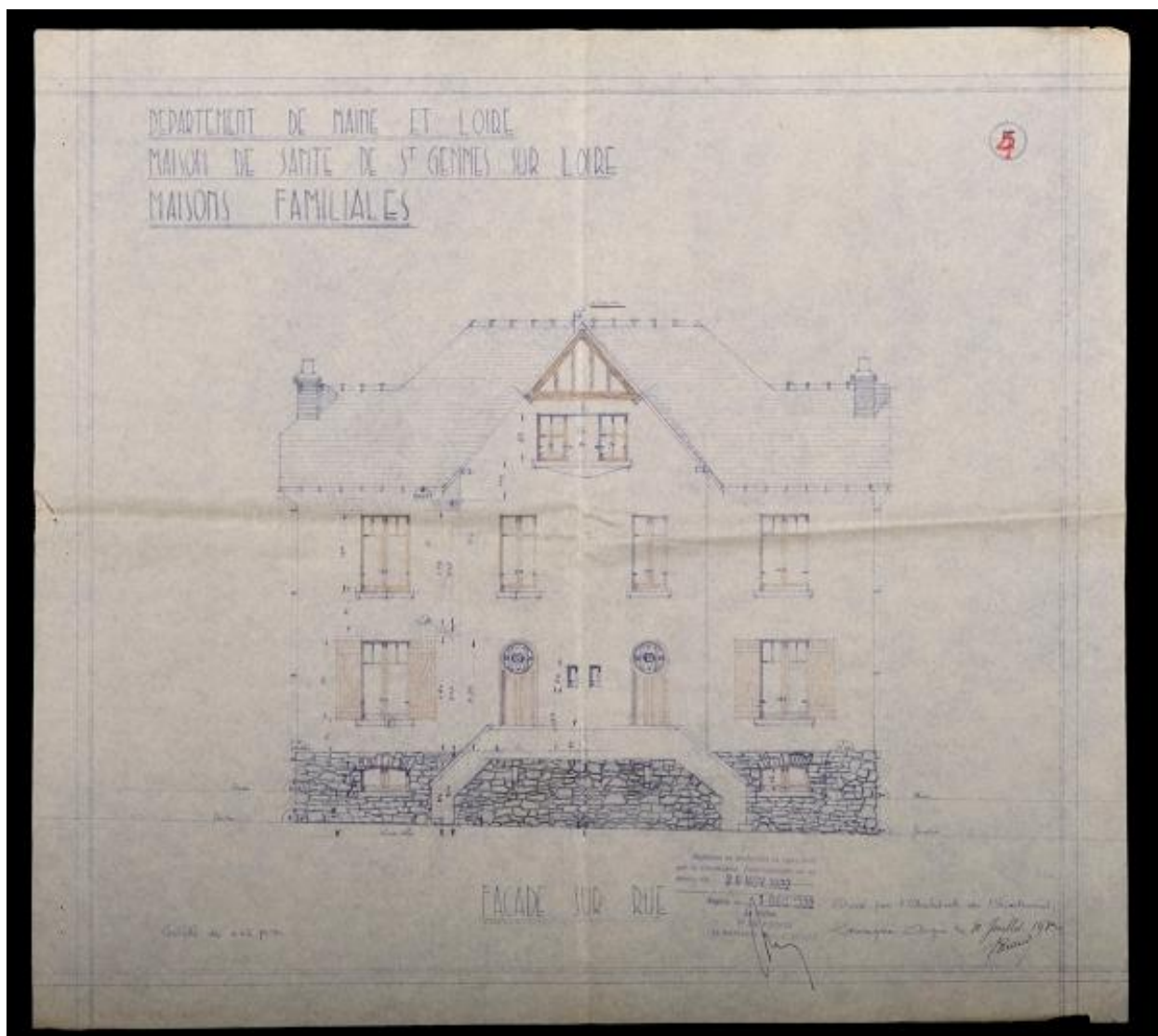
Maisons familiales. Façade sur rue, par Ernest Bricard. Juillet 1932. (Archives départementales de Maine-et-Loire, 4 N).
