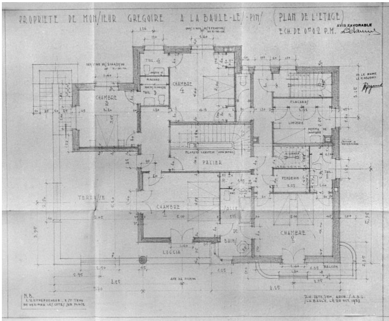
Plan au 1/50e de l'étage de la villa Aktina.
