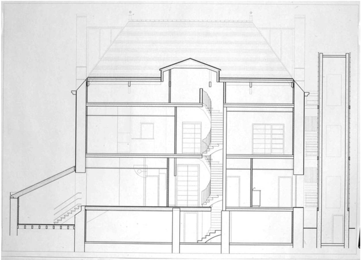
Coupe longitudinale.
