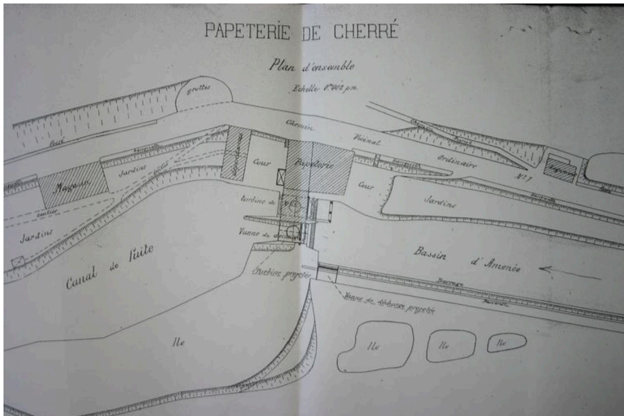
Plan général de la papeterie et du barrage de Cherré.
