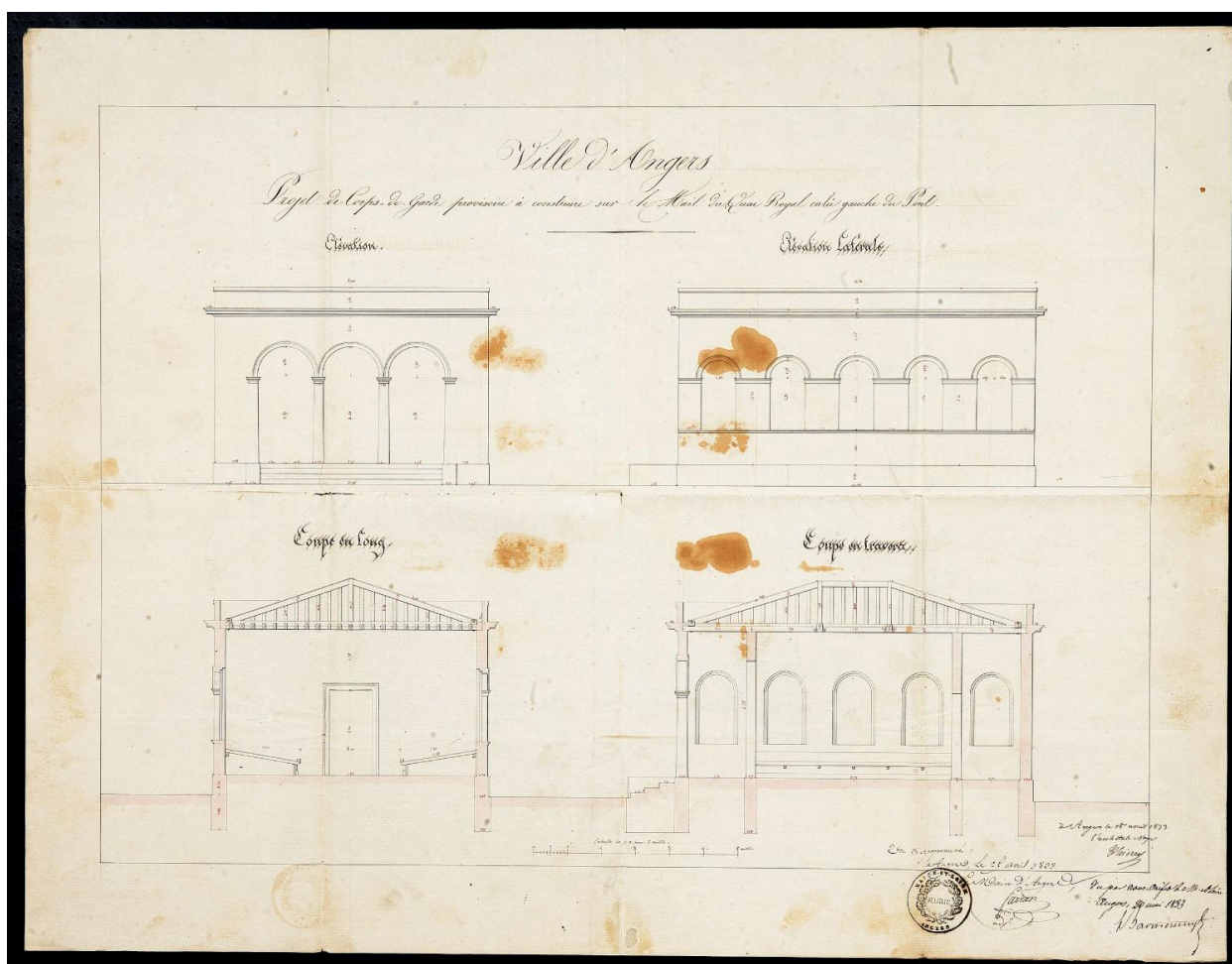
Ville d'Angers. Projet de corps de garde provisoire à construire sur le mail du quai Royal culée gauche du pont (deuxième projet proche de l'état réalisé), élévation antérieure et latérale, coupes transversale et longitudinale, par B. Thierry, 1833.
