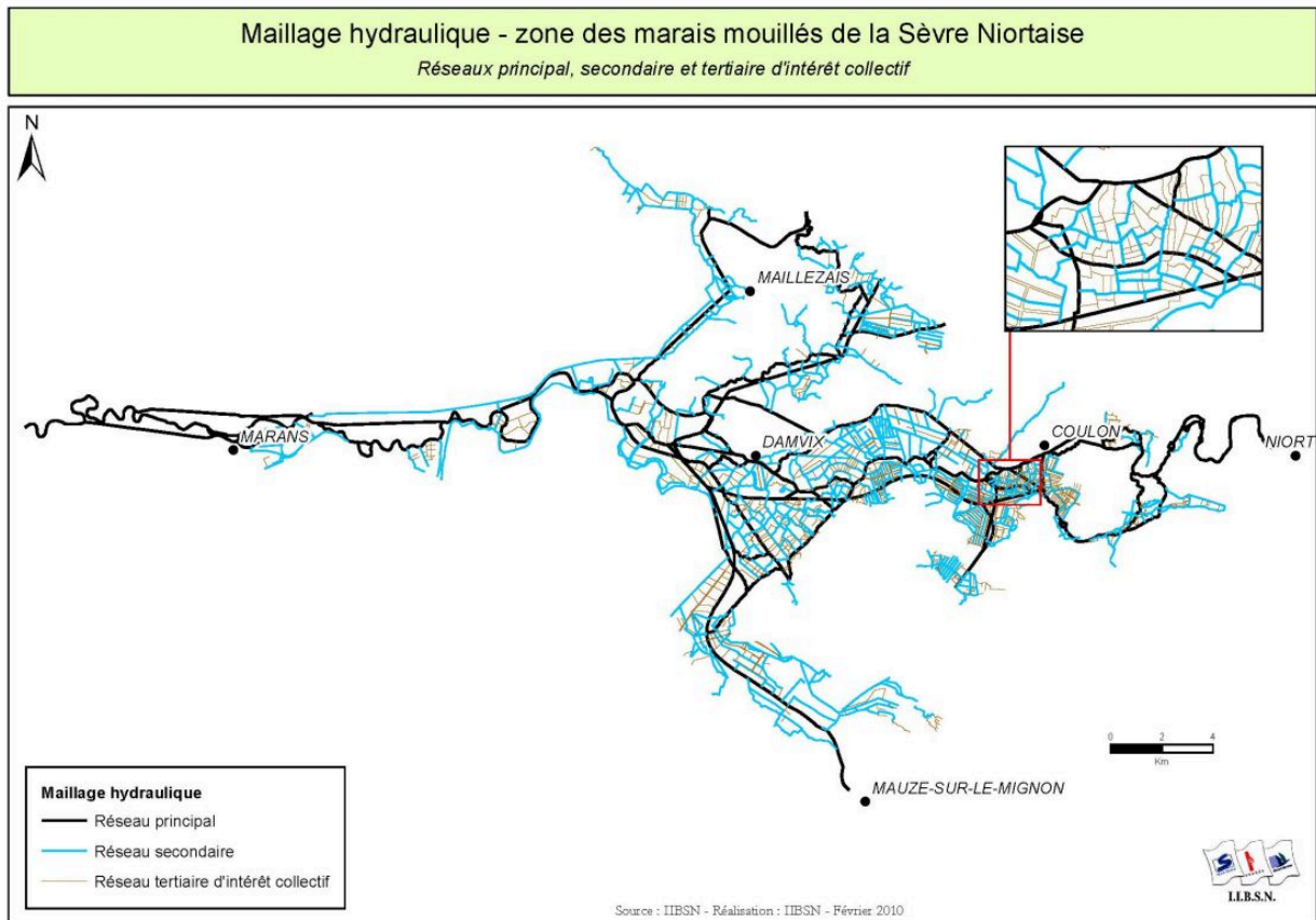
Carte du maillage hydraulique des marais mouillés du Marais poitevin (source : I.I.B.S.N.).
