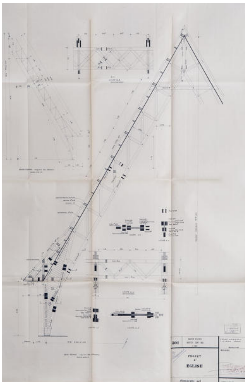
Coupe de la charpente de l'église, 1963.
