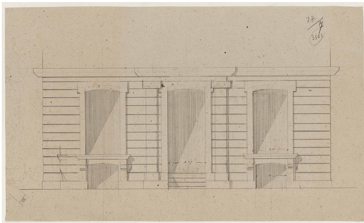
Maison d'habitation appartenant à Monsieur Broutelle. Élévation de fenêtres et de la porte d'entrée du rez-de-chaussée. 1862. (Archives départementales de Maine-et-Loire, 90 J 3996).
