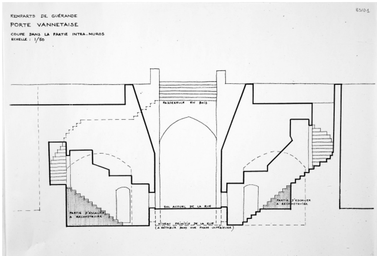
Coupe longitudinale.
