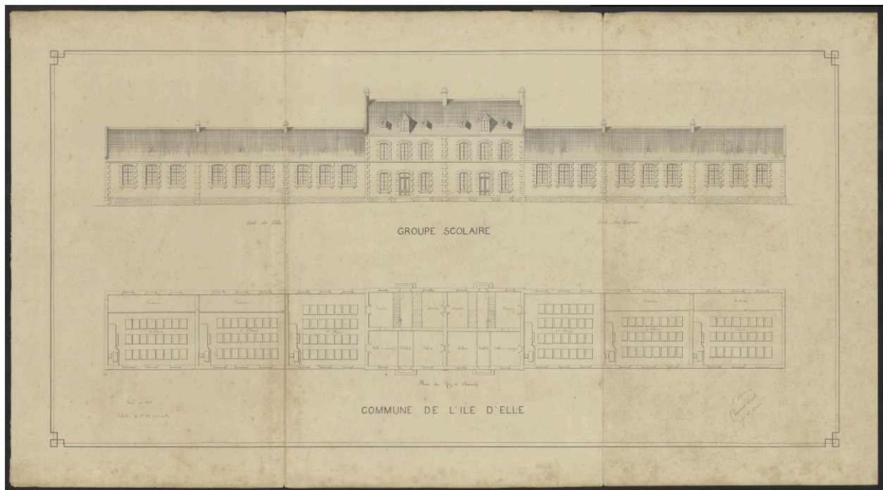
Élévation et plan du groupe scolaire.
