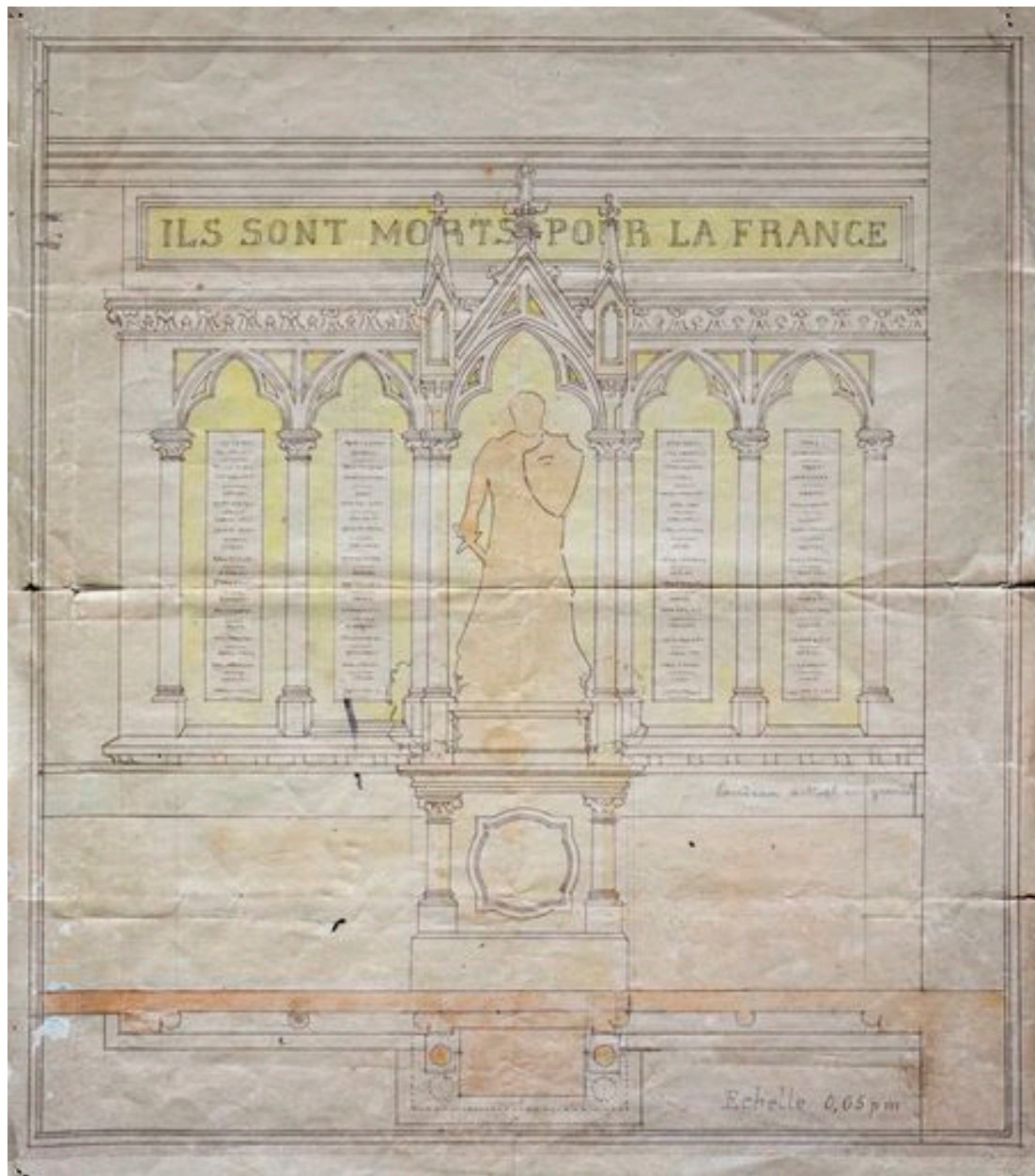
Projet définitif des architectes nantais J et P Bougoüin, élévation et plan au sol.
