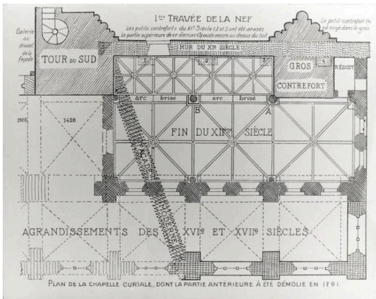
Plan de la chapelle curiale, dont la partie antérieure a été démolie en 1791 : reconstitution chronologique, par Louis de Farcy. Relevé imprimé, [début 20e siècle]. In : FARCY, Louis de : "Monographie de la cathédrale d'Angers", Angers : Josselin, A. Bruel, Paris, Bruges : Desclée, De Brouwer, 1910, vol. 1.
