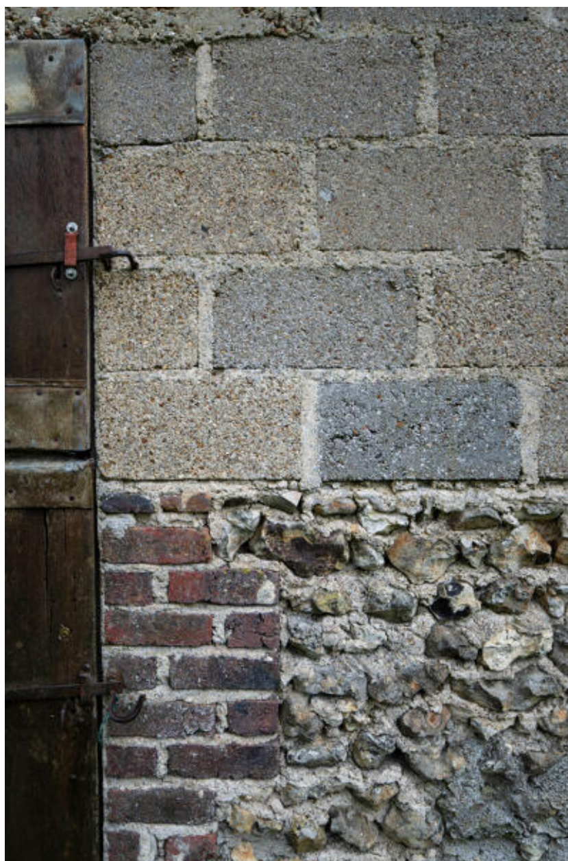
Grange-étable : détail.
