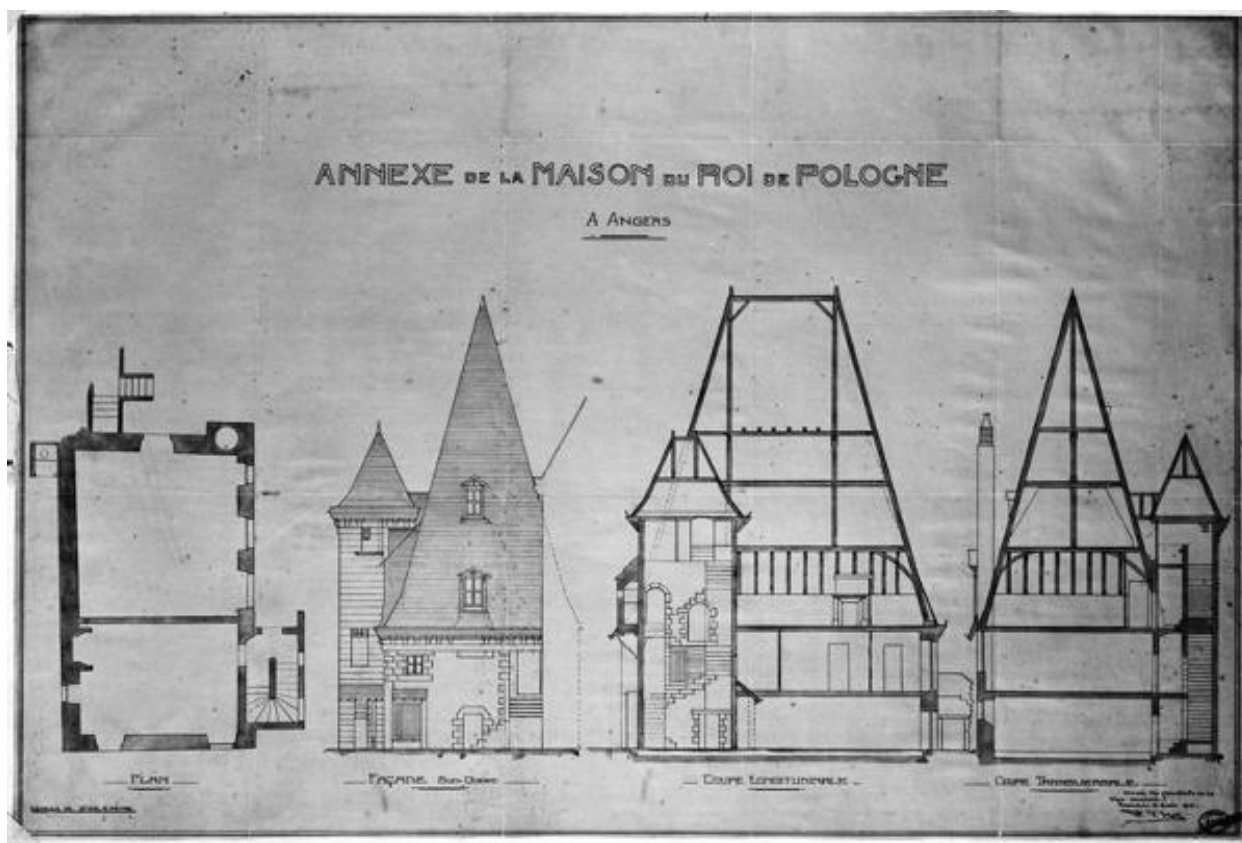
Corps de logis annexe : plan du rez-de-chaussée, coupes et élévation, éch. 1:50e, par R. Brot, 1914. (Médiathèque de l'Architecture et du Patrimoine ; 47070).
