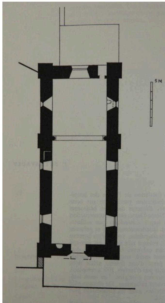
Plan de l'église de Puyravault.
