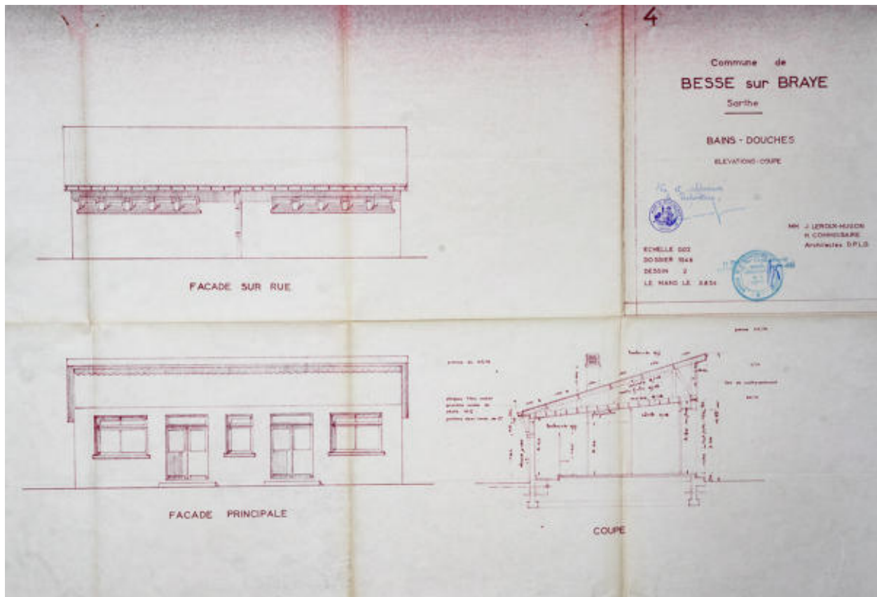
Elévations et coupe des bains-douches.
