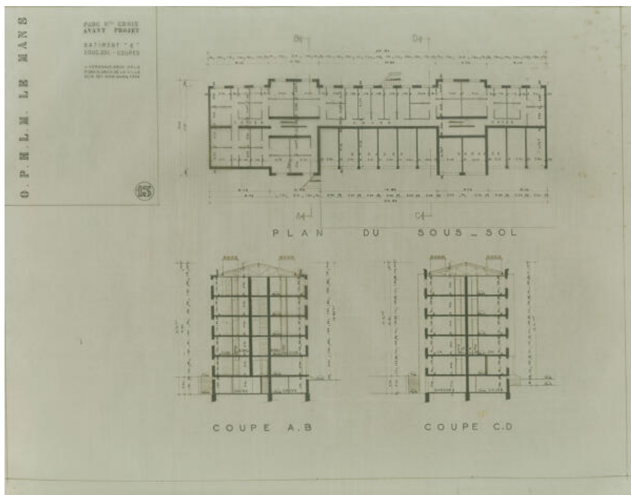
Plan des cellules et de la distribution du bâtiment E.
