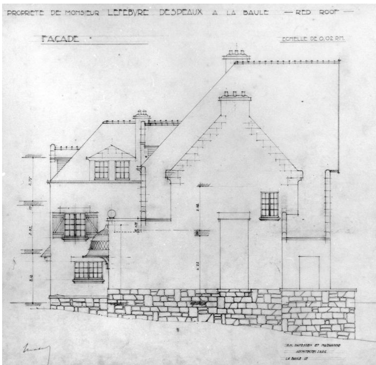
Façade ouest au 1/50e de la villa Red-Roof pour M. Lefebvre Despeaux en 1926.
