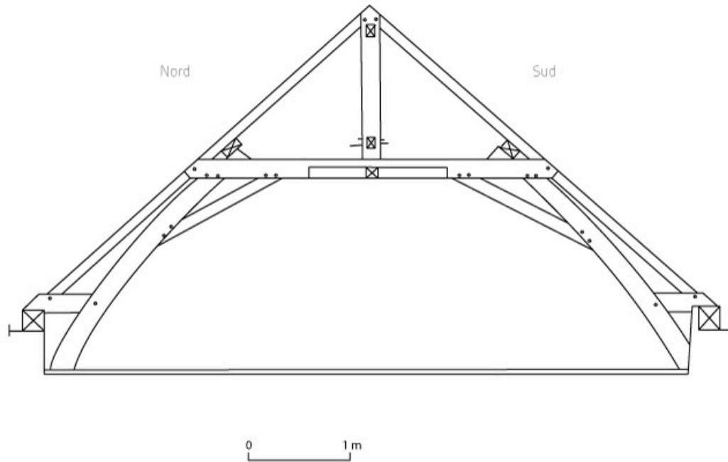
VAIGES - Les Guetteries COUPE TRANSVERSALE D'UNE FERME DE LA CHARPENTE SELON AA
