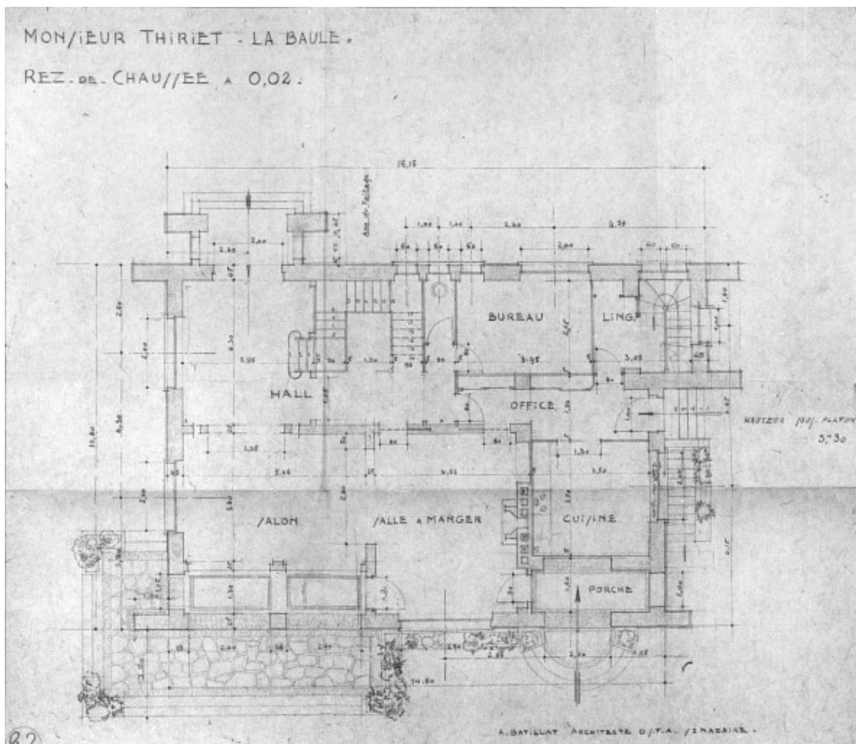
Plan du rez-de-chaussée au 1/50e de la villa Blanche dressée pour M. Thiriet.
