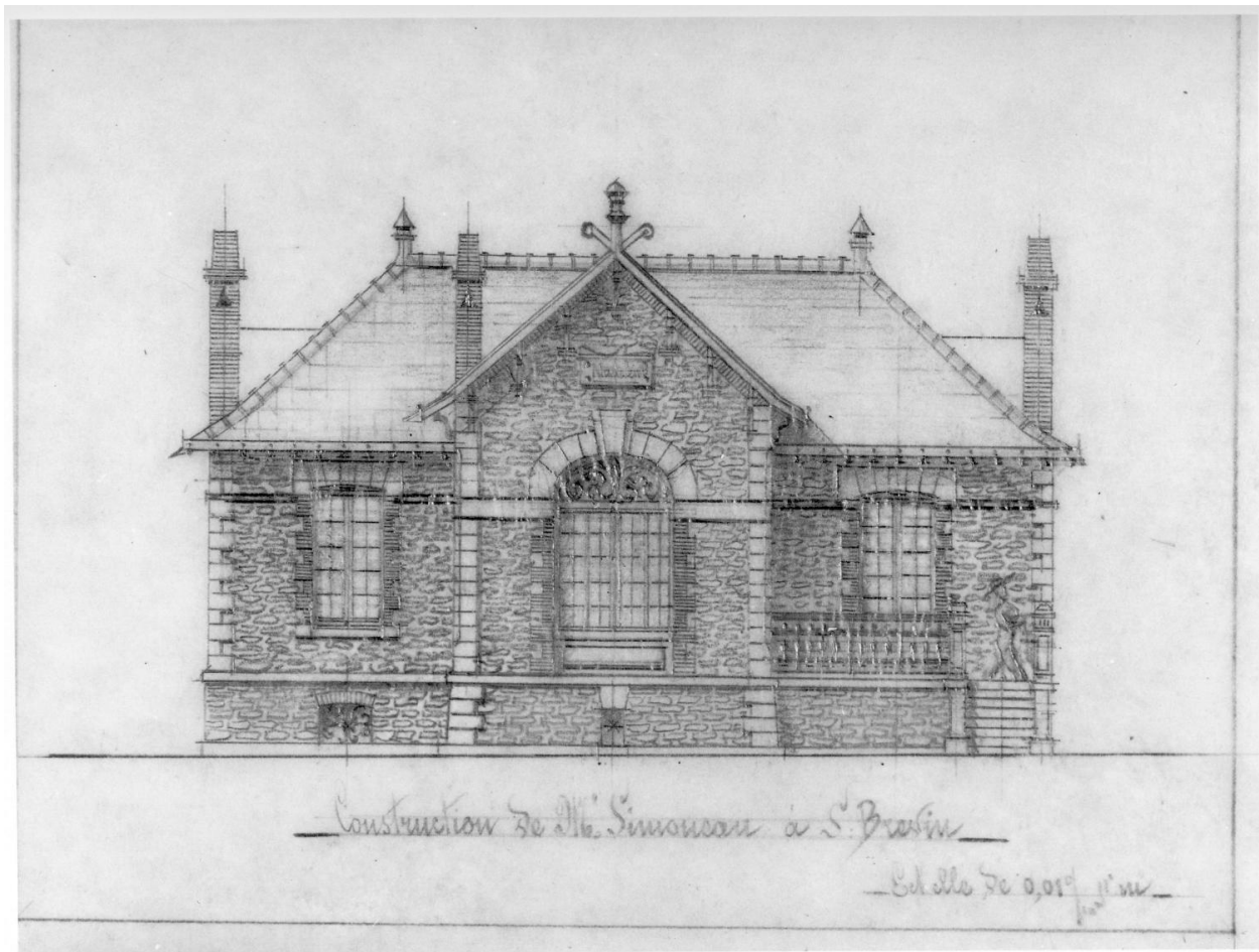
"Construction de Monsieur Simoneau à Saint-Brevin", élévation antérieure, au 1:50e.
